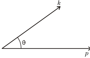
Рис.4. Направление полета квазичастицы (угол \theta ) отсчитывается от импульса частицы p .
