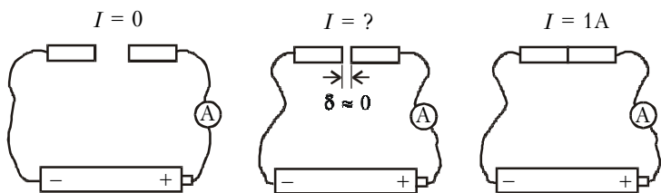
Рис.1. При большом зазоре между проводниками ток равен нулю, при контакте проводников в цепи течет ток, например 1 А. До какого расстояния d нужно сблизить два проводника, чтобы появился заметный электрический ток?
